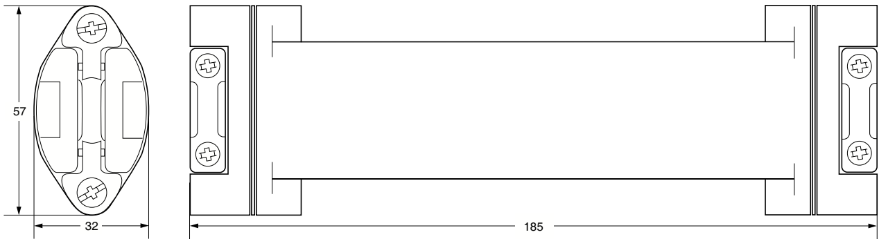
尺寸 (mm)
