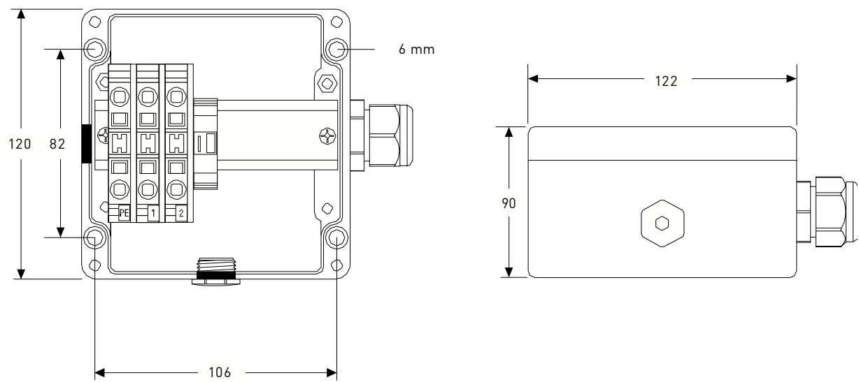
尺寸 (mm)
